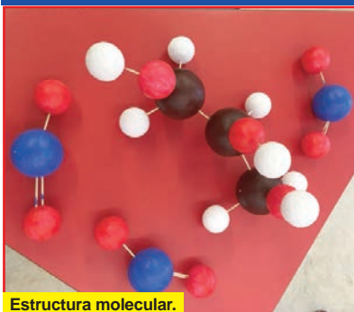
Estructura molecular.
